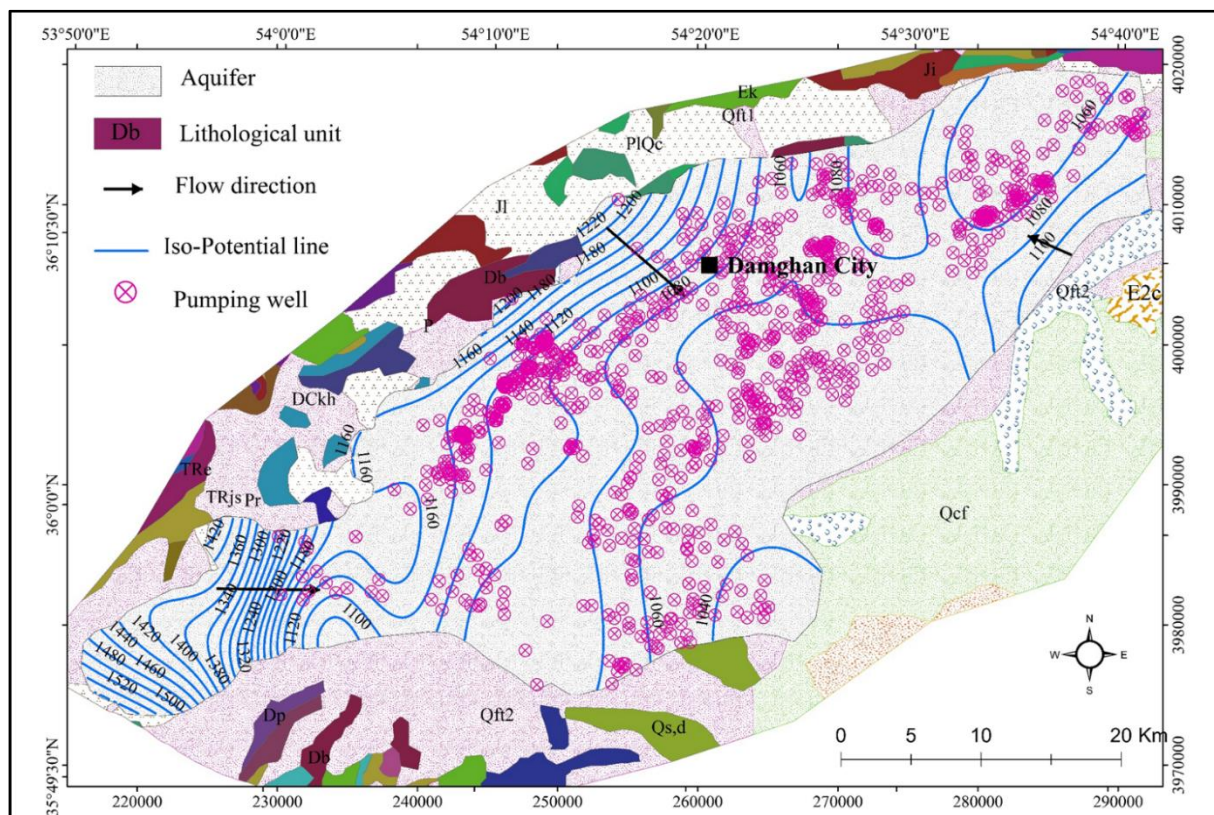
شکل ۱. واحدهای زمین‌شناسی، خطوط هم‌پتانسیل آب زیرزمینی و موقعیت آبخوان دامغان. فلش‌های قرمز جهت جریان آب زیرزمینی را نشان می‌دهند.
